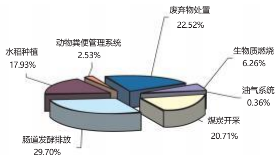
图 2.4 1994 年中国甲烷排放源及构成
