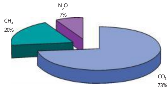
图 2.1 1994 年中国温室气体排放构成
